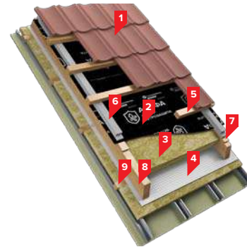
Рис. 6. Строение кровельной системы TH-ЛЮКСАРД Мансарда
