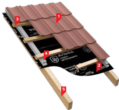
Рис. 5. Строение кровельной системы TH-ЛЮКСАРД Классик
