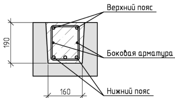
Рис. А.1. Элементы армирования балки в U-образном блоке
